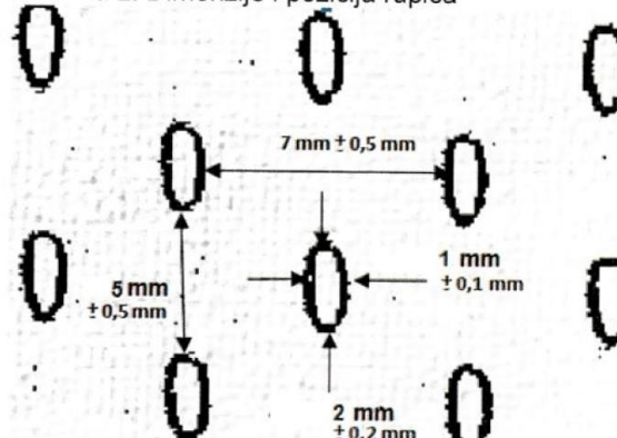
Slika 2. Dimenzije i pozicija rupica
